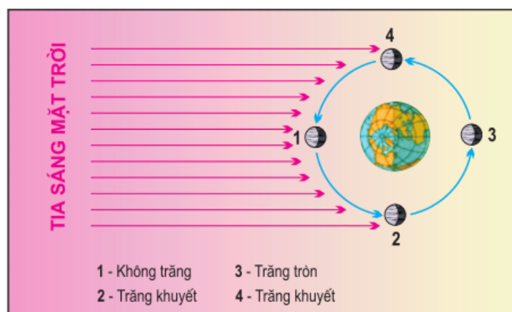
Hình 16.1 - Chu kỳ tuần trăng
