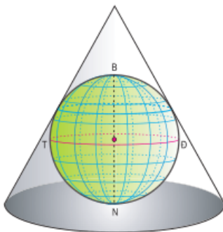
Hình 1.5a - Phép chiếu hình nón đứng
