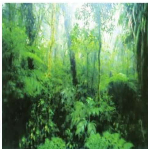
Hình 19.10 - Rừng nhiệt đới ẩm
