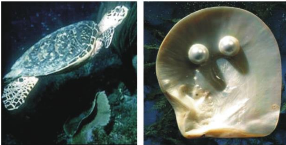
Hình 29.4 – Đồi mồi và trai ngọc
