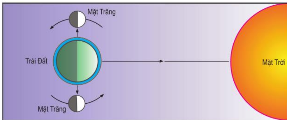
Hình 16.3 – Vị trí của Mặt Trăng vào các ngày “triều kém” (dao động thủy triều nhỏ nhất)
