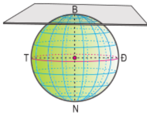
Hình 1.3a – Phép chiếu phương vị đứng
