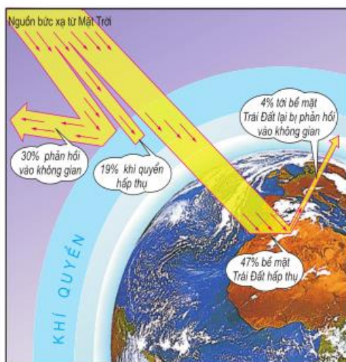
Hình 11.2 – Phân phối bức xạ mặt trời
