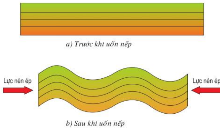
Hình 8.1 – Hiện tượng uốn nếp
