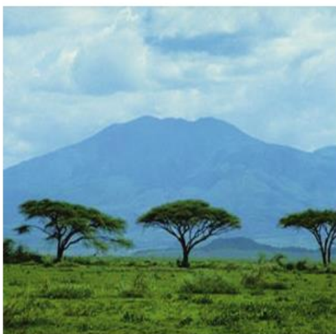
Hình 19.9 - Xavan
