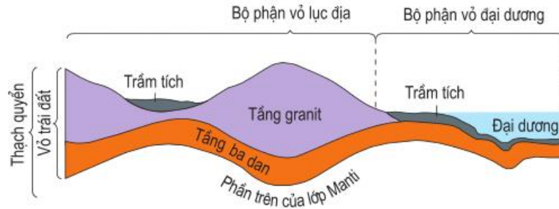
Hình 7.2 – Lớp vỏ Trái Đất. Thạch quyển
