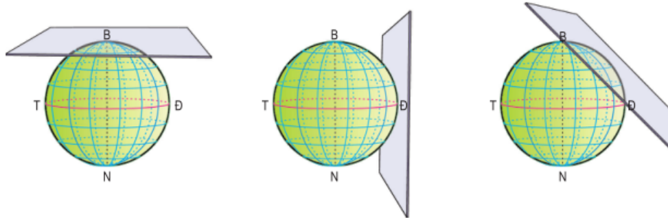
a - Phép chiếu phương vị đứng b - Phép chiếu phương vị ngang c - Phép chiếu phương vị nghiêng
