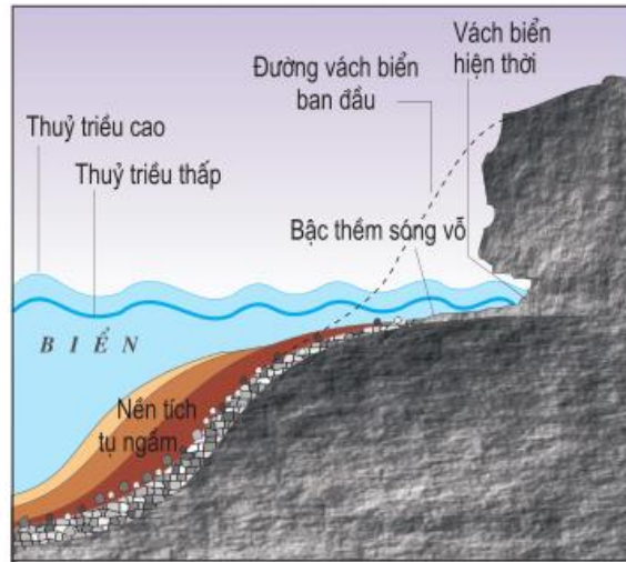
Hình 9.6 – Vách biển và bậc thềm sóng vỗ
