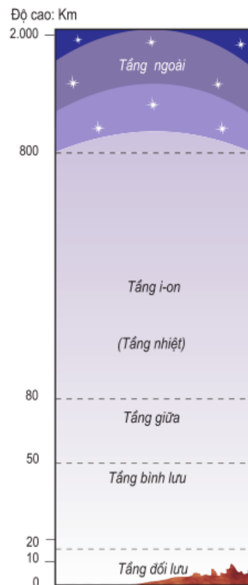
Hình 11.1 – Các tầng khí quyển
