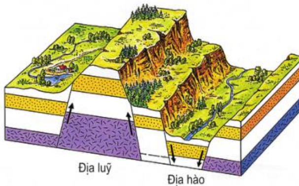
Hình 8.3 – Địa lũy và địa hào
