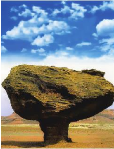
Hình 9.5 – Nấm đá
