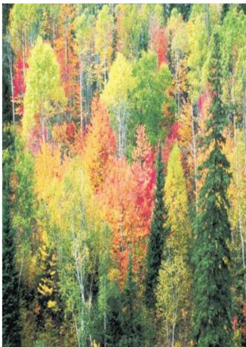
Hình 19.7 - Rừng cận nhiệt ẩm
