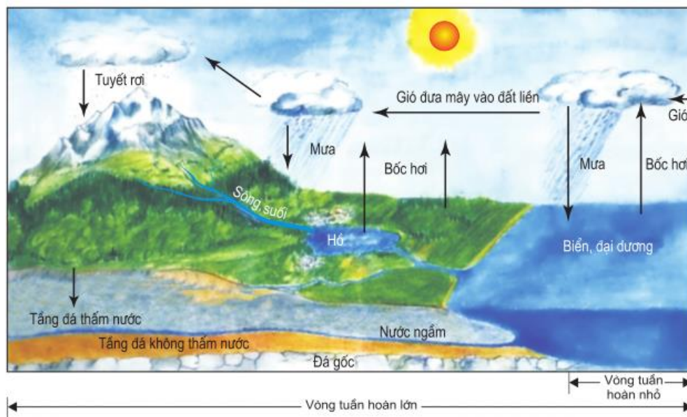
Hình 15 – Sơ đồ tuần hoàn của nước
