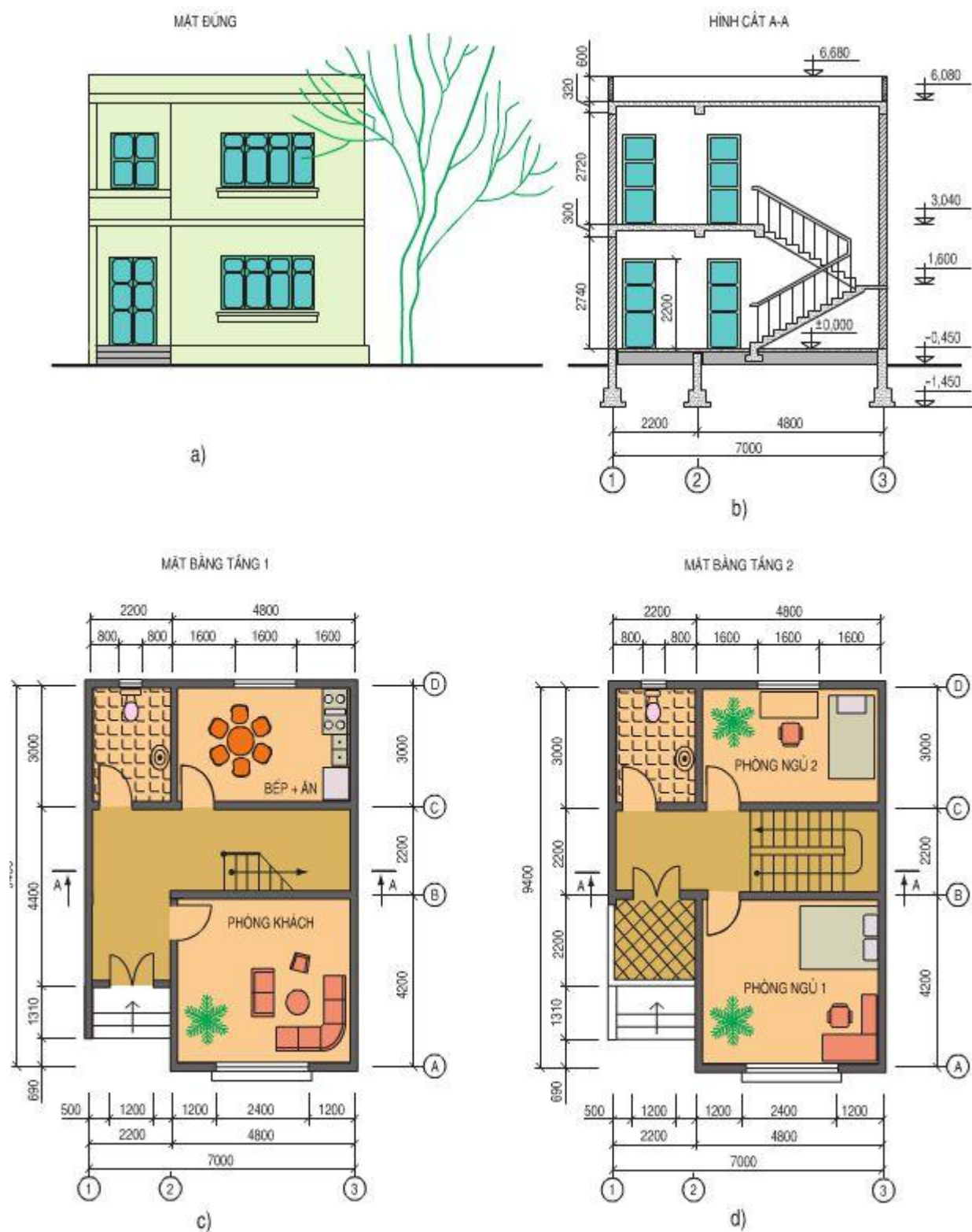
Hình 11.2. Bản vẽ nhà ở hai tầng
