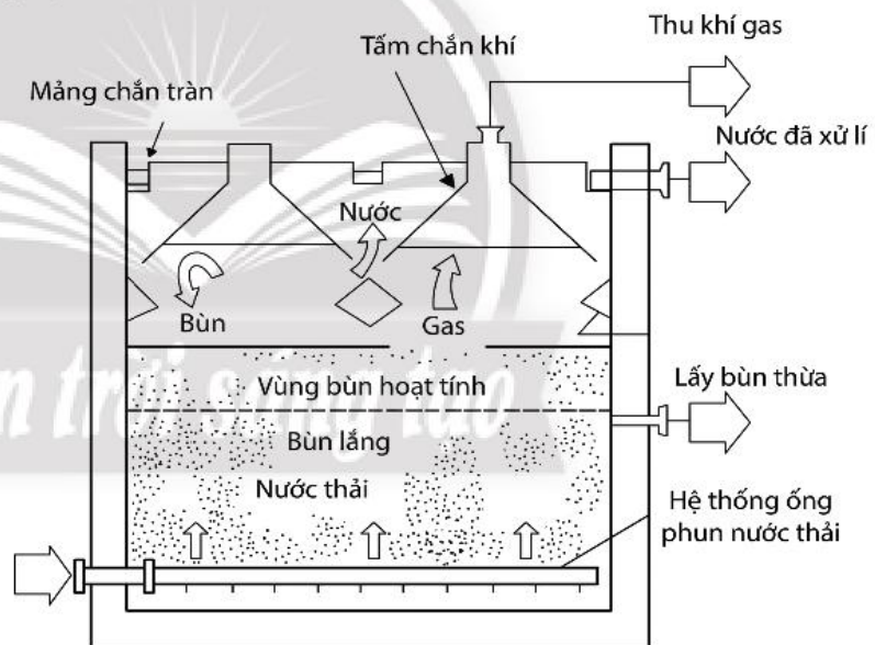
Hình 27.6. Xử lý nước thải bằng bể UASB
