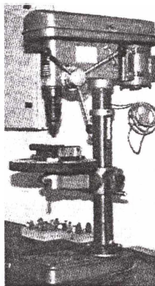
Hình 14.1. Máy khoan bàn
