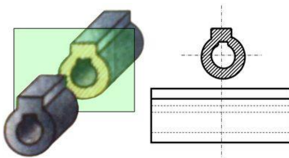
Hình 4.5. Hình biểu diễn mặt cắt rời của vật thể
