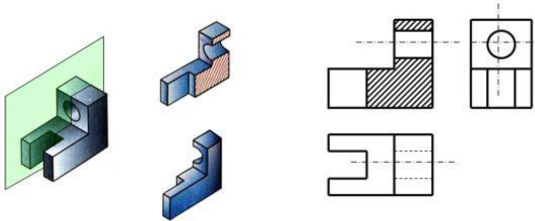
Hình 4.6. Hình cắt toàn bộ
