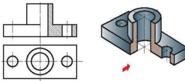
Hình 4.7 Hình cắt một nửa
