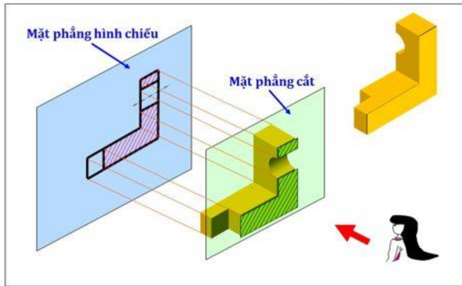
Hình 4.1. Xây dựng hình cắt và mặt cắt
