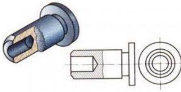
Hình 34.8. Hình cắt cục bộ
