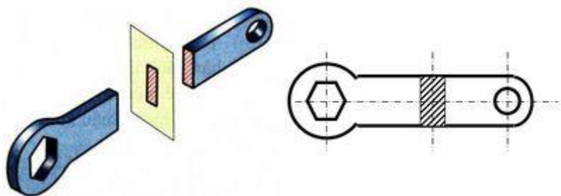
Hình 4.4. Hình biểu diễn mặt cắt chập của vật thể
