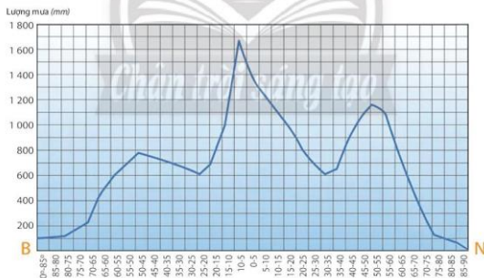
Hình 10.1. Phân bố lượng mưa theo vĩ độ
