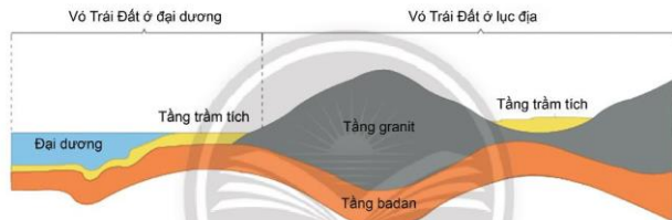
Hình 4.2. Lớp vỏ Trái Đất
