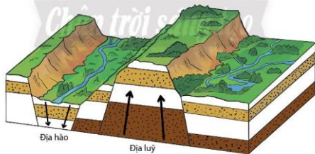
Hình 6.4. Địa hào và địa lũy
