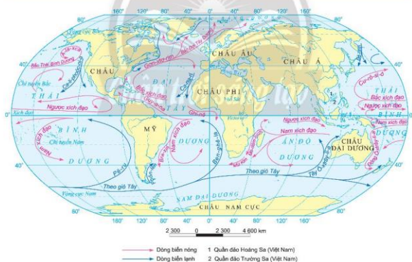
Hình 13.4. Dòng biển trong các đại dương
