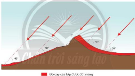
Hình 8.2. Nhiệt độ thay đổi theo độ dốc và hướng phơi của sườn núi
