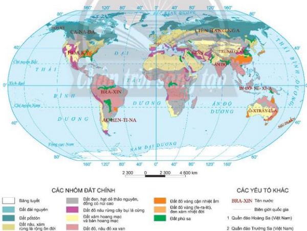
Hình 16.1. Các nhóm đất chính trên thế giới
