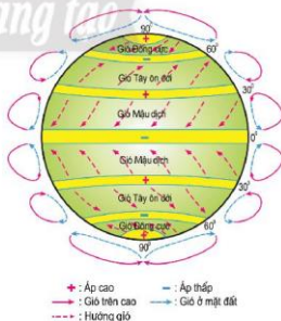
Hình 9.1. Các đai khí áp và gió trên Trái Đất
