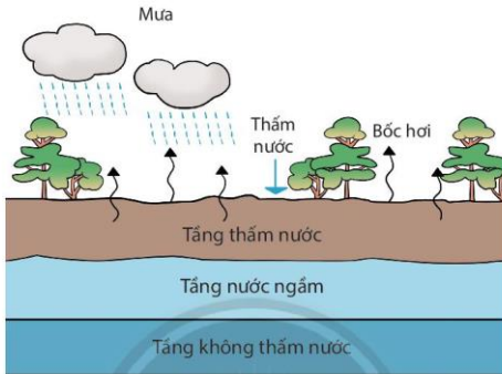
Hình 12.2. Sơ đồ cấu trúc nước ngầm
