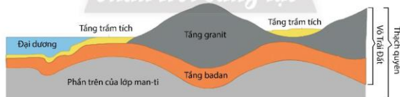
Hình 6.1. Thạch quyển
