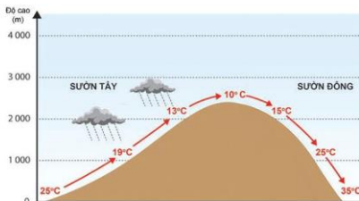
Hình 9.3. Quá trình hình thành gió phơn
