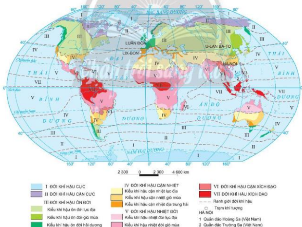
Hình 11.1. Các đới khí hậu trên Trái Đất
