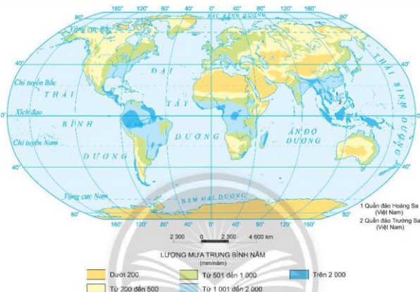
Hình 10.2. Phân bố lượng mưa trung bình năm trên các lục địa
