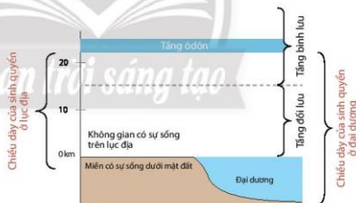
Hình 15. Giới hạn của sinh quyển
