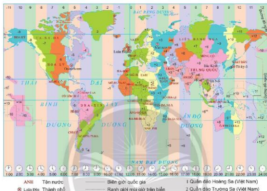
Hình 5.2. Các múi giờ trên Trái Đất
