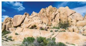
Hình 7.1. Sự nứt vỡ của đá do nhiệt độ thay đổi đột ngột (Ca-li-phoóc-ni-a – Hoa Kỳ)
