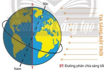
Hình 5.1. Sự luân phiên ngày, đêm
