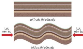
Hình 6.2. Hiện tượng uốn nếp
