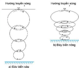
Hình 13.1. Chuyển động của sóng biển
