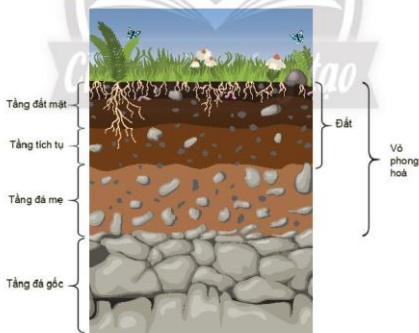
Hình 14.1. Đất và lớp vỏ phong hoá
